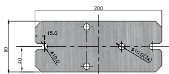
Suporte teto (TE) (Ceiling support)
