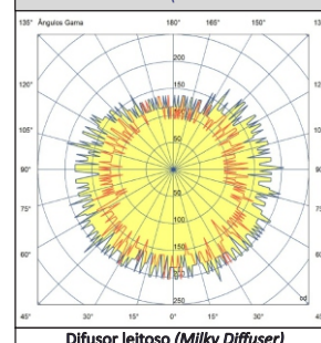
Curva fotométrica(Photometric Curve)
