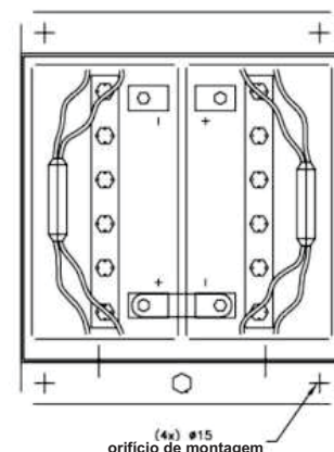
VISTA DO PLANO DO BANCO DE BATERIAS
