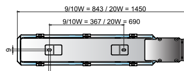
Suporte Z (ZZ) (Support ZZ)
