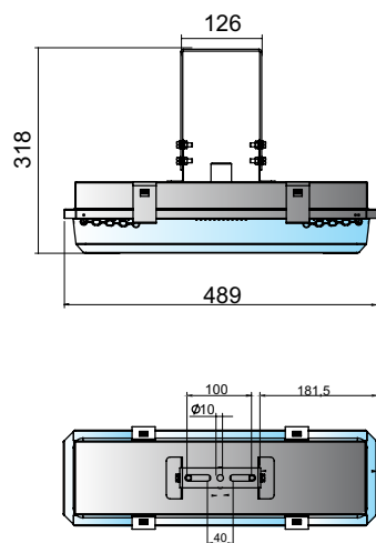
Fixação por Eletroduto com Alça Ajustável (T □) (Attachment by conduit) T3 - 3/4" T7 - 1/2"
