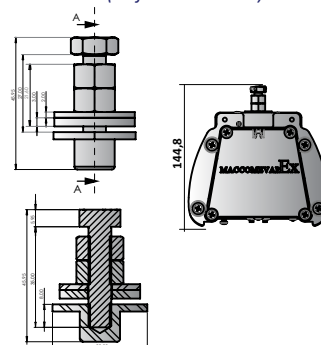
Suporte Regulável- (SR) (Adjustable stand)
