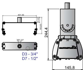
Suporte Pendente para Fixação de Eletroduto-(D□) (Support pending for Attachment of conduit)
