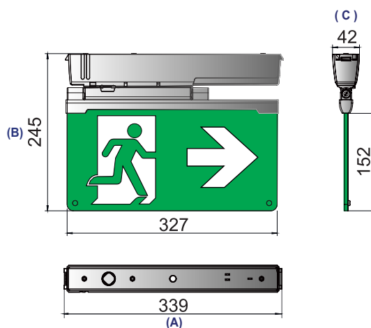
DESENHO DIMENSIONAL (mm) (Dimensional Drawing)
